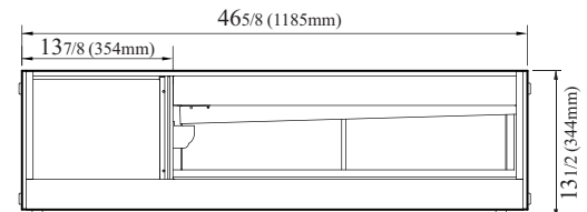
SAS-50L-N
